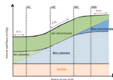
Figure 1: Schéma des courbes de retrait avec les 4 points du modèle XP (MS, ML, AE, SL), les 3 pentes (K) et les différents volumes fonctionnels de la porosité. Source : Lamy (2009), modifié.
