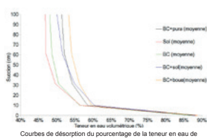
Courbes de désorption du pourcentage de la teneur en eau de BC+pura, Sol, BC, BC+sol et BC+boue
