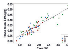
Figure 4: Droite de régression de la teneur en eau au point MS en fonction de la teneur en Corg.
