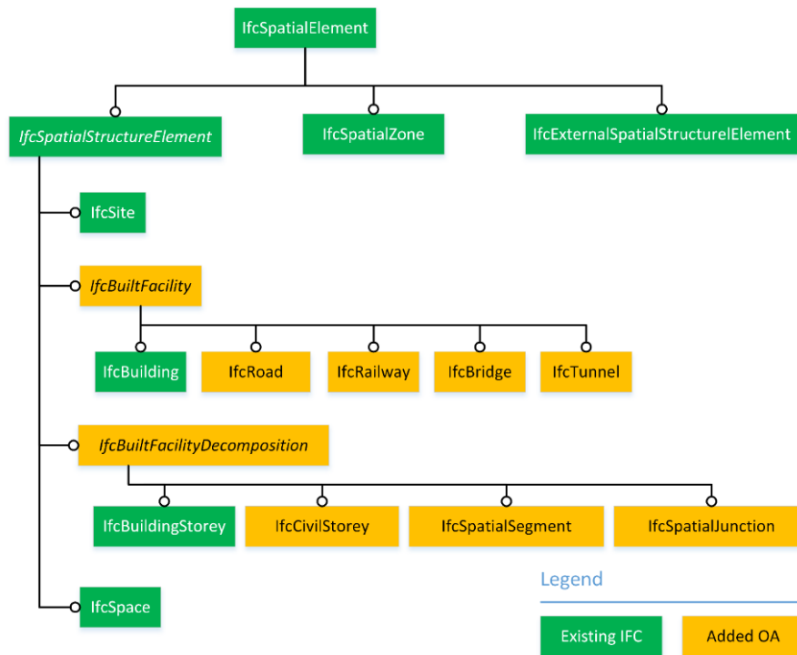
Bild 6: Die überarbeitete Struktur der IFC in der Version 5 [4]
