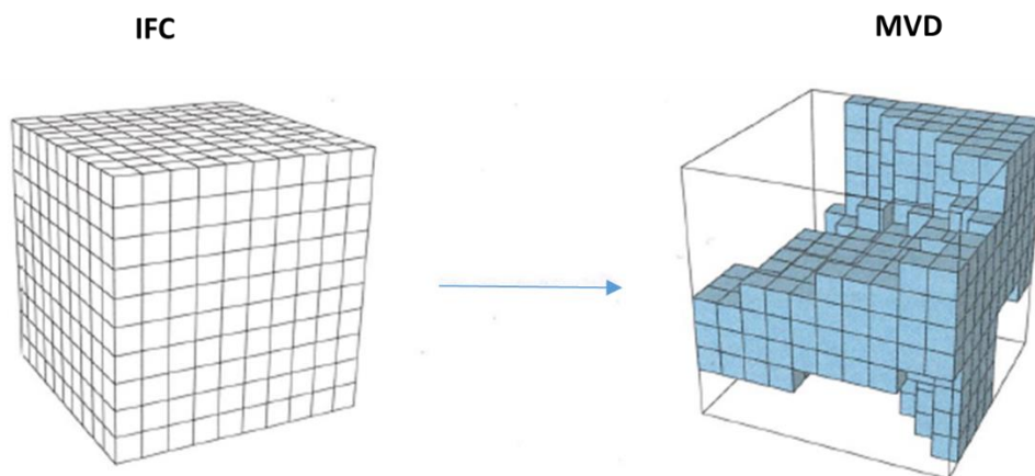
Bild 5: MVD – eine Teilmenge der IFC [2]
